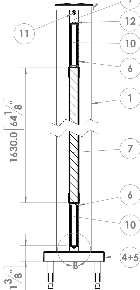
SECTION B-B SCALE 1 : 4
