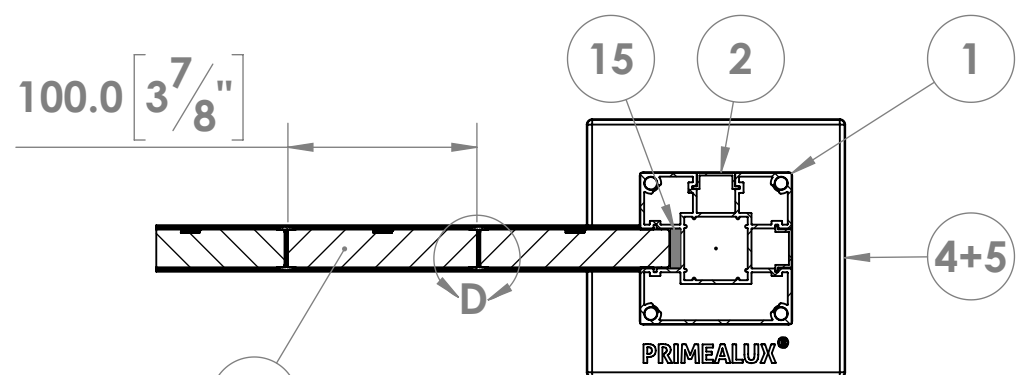
SECTION A-A SCALE 1 : 4
